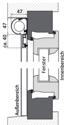
Montage auf dem Fensterrahmen (vertikal)
