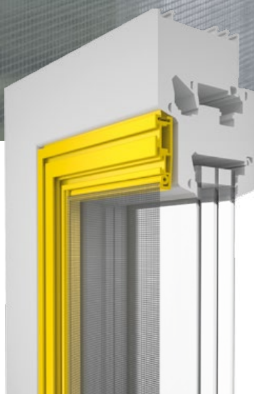
SP-F pour fenêtres avec débord et goupille à ressort
