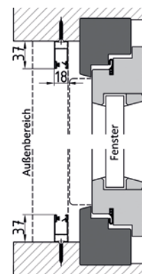
Montage in der Laibung
