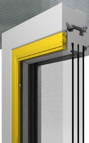
SP-F für flächenversetzte Fenster mit Federstift
