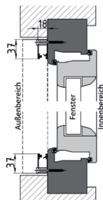
Montage auf dem Fensterrahmen (horizontal)
