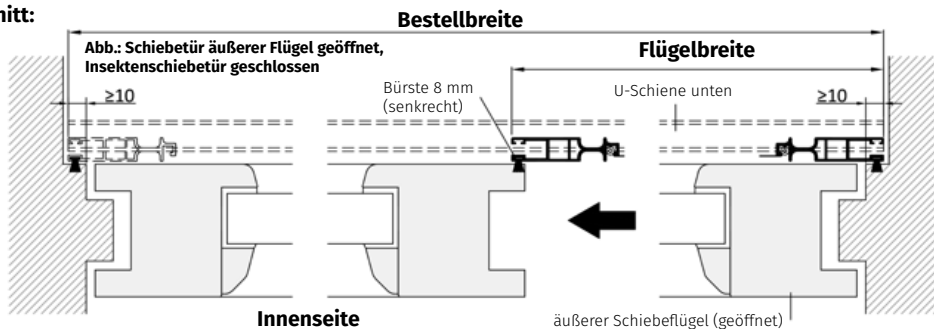
Abb.: Hebe-Schiebetür
