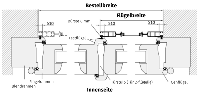
Horizontalschnitt V1: für 2-flügelige Stulp-Tür
