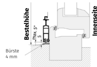
Vertikalschnitt V2: T-Bodenschiene
