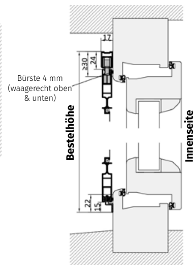
Vertikalschnitt V2: T-Bodenschiene
