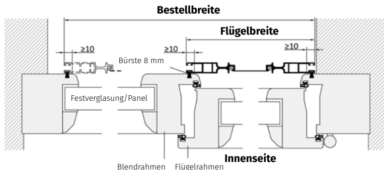
Horizontalschnitt V2: für 1-flügelige Tür mit feststehendem Teil
