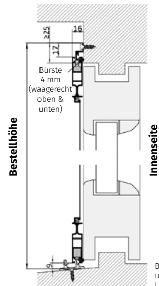
Vertikalschnitt V1: U-Profil unten bis 10° geneigt möglich
