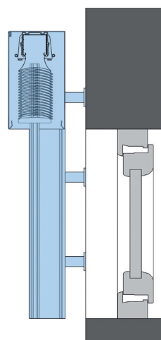
auf der Fassade mit Abstandshaltern
