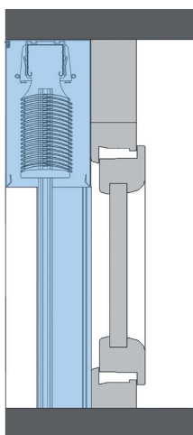
in der Laibung als sichtbarer Kasten
