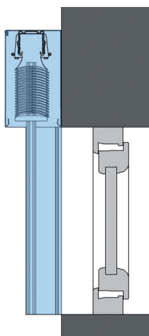
auf der Fassade
