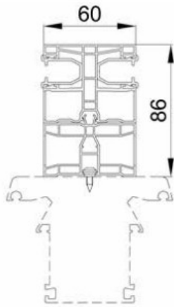
DF K 74 (Raffstore)
