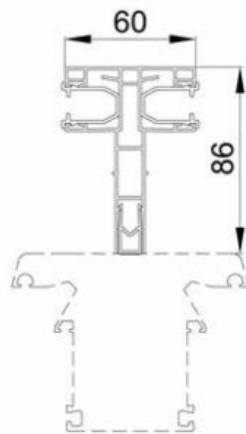
DF A 74 (Raffstore)
