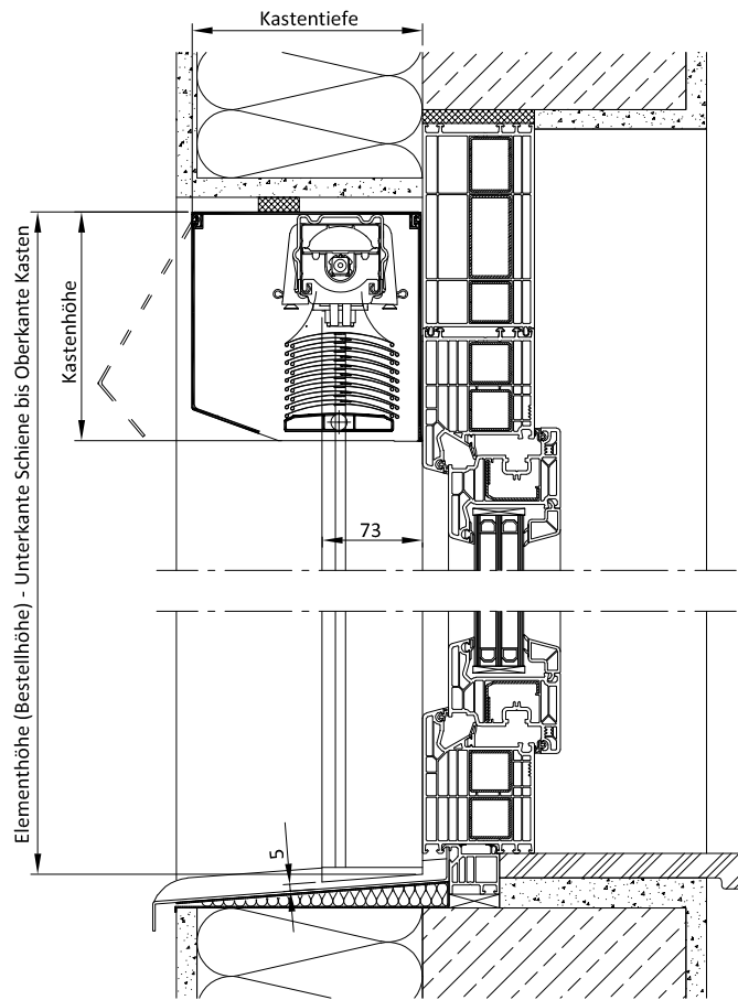
Vorbauraffstore 20° Kasten Revision vorn Kastengröße 165 Alu-Führungsschiene
