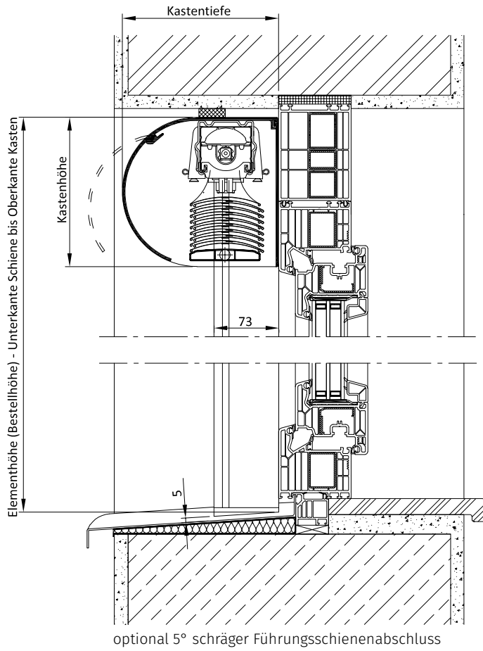
Vorbauraffstore Rundkasten Kastengröße 165 Alu-Führungsschiene
