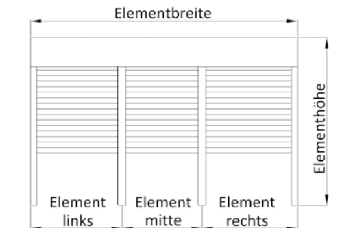
(V6) 3er Kombination mit Einzelführungsschienen (mittig)
