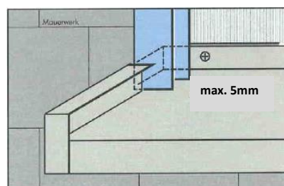
Bild 2: Ausklinkung des Bordprofils für den Einstand der Führungsschiene (in unverputztem/ungedämmtem Zustand, Isometrie)
