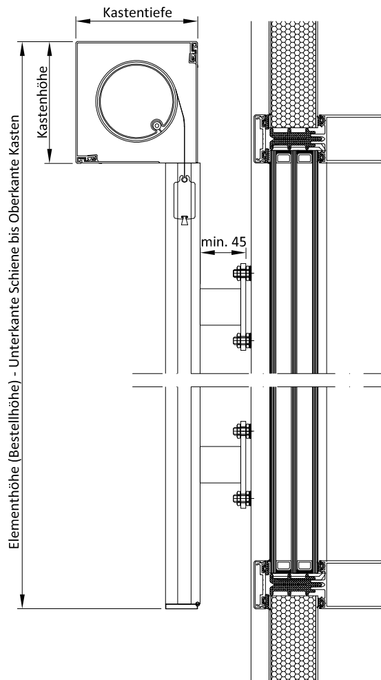
Vorbaukasten ZipTex - Aufgeständert 90° Kasten Kastengröße 100 Alu-Führungsschiene
