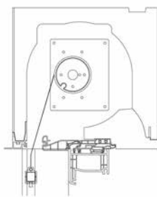
ZIPTEX – REVISION AUßEN
