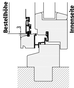
Variante 2: Wetterschenkel am Blendrahmen
