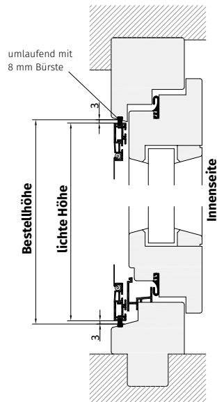
Variante 2: Wetterschenkel am Blendrahmen
