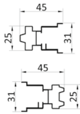
Griffprofil und Gegenstück
