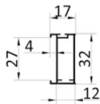
Rahmenprofil
