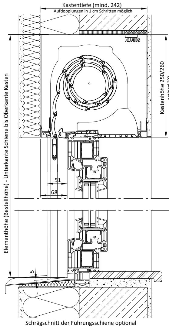
AK-FLEX.2 Revision innen Kastengröße 270x260 PVC-Führungsschiene Führungsschienenschrägschnitt
