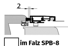
im Falz SPB-8 Standard: Breite: BRÜL abzgl. 4 mm Höhe: BRÜL abzgl. 4 mm
