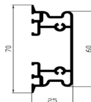
Griffleiste RT 50
