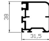
Rahmenprofil RT-50
