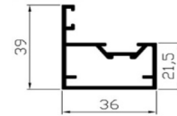
Rahmenprofil RT-50
