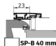
SP-B 40 mm Standard: Breite: BRÜL + 46 mm Höhe: BRÜL + 50 mm
