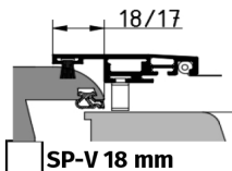
SP-V 18 mm Standard: BRÜL + 36 mm (Breite und Höhe)
