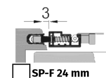
SP-F 24 mm Standard: Breite: BRÜL abzgl. 6 mm Höhe: BRÜL abzgl. 6 mm
