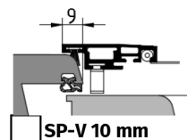
SP-V 10 mm Standard: BRÜL + 18 mm (Breite und Höhe)
