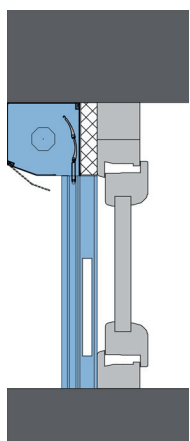
Vorbaurollladen
