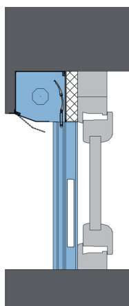
Putzträgerrollladen
