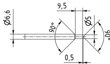
Bohrbild für Federscharnier (Bohrschablone)
