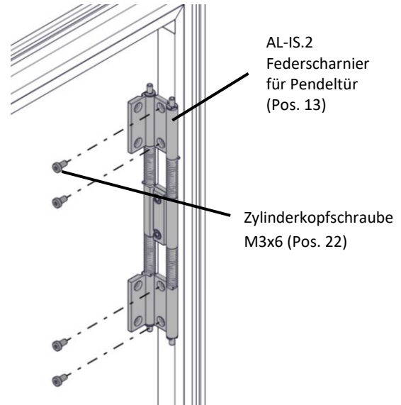
Flügel an Rahmen befestigen (Federscharnier f. PT)
