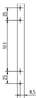
Bohrbild für Federscharnier (Bohrschablone)
