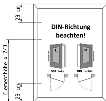
Maße für Bohrbild mittig
