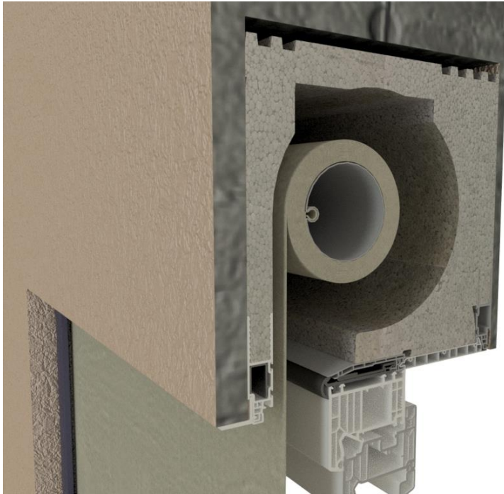
Bild 1: Mit dem AK-Flex mit integriertem ZipTex kombiniert Alukon einen ins Mauerwerk integrierten Kasten mit textilem Sonnenschutz.
