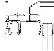
Führungsschiene A74 + A76
